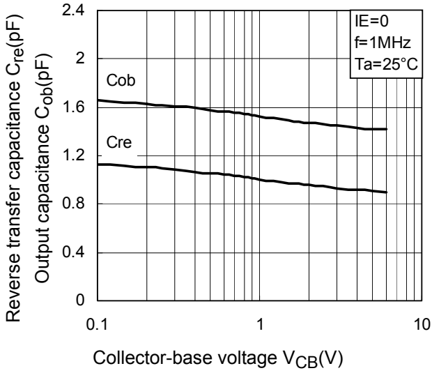
C_{re}, C_{ob}-V_{CB}
